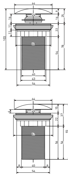
D 501 ДОННЫЙ КЛАПАН Размер: 64 x 64 x 103 мм
