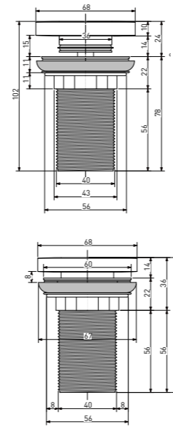
D 504 ДОННЫЙ КЛАПАН Размер: 68 x 68 x 102 мм
