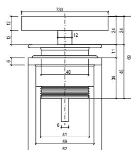
D 604 ДОННЫЙ КЛАПАН Размер: 67 x 67 x 65 мм
